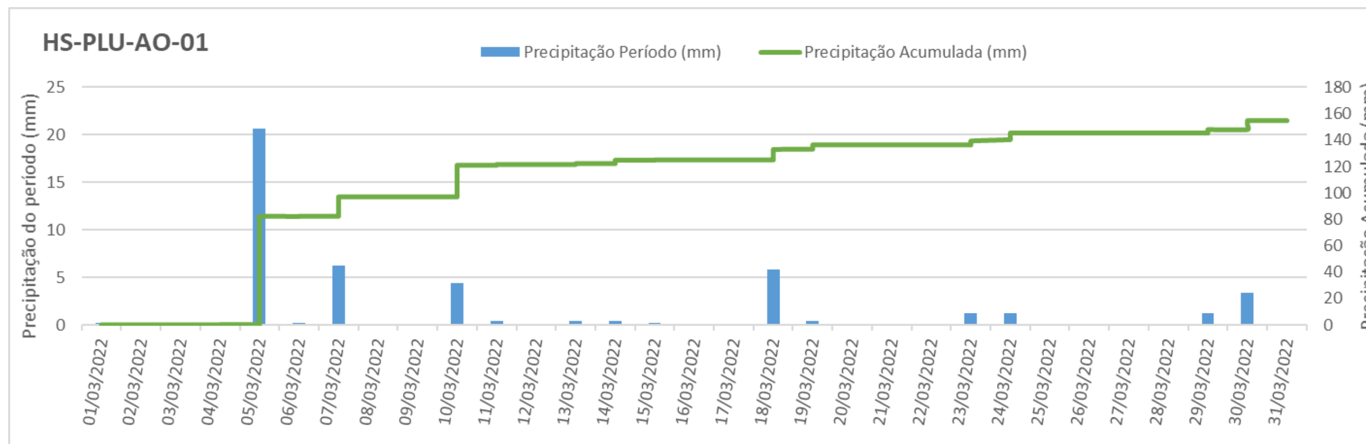
Figura 9 – Precipitação (mm) na Estação Arroio do Ouro.
