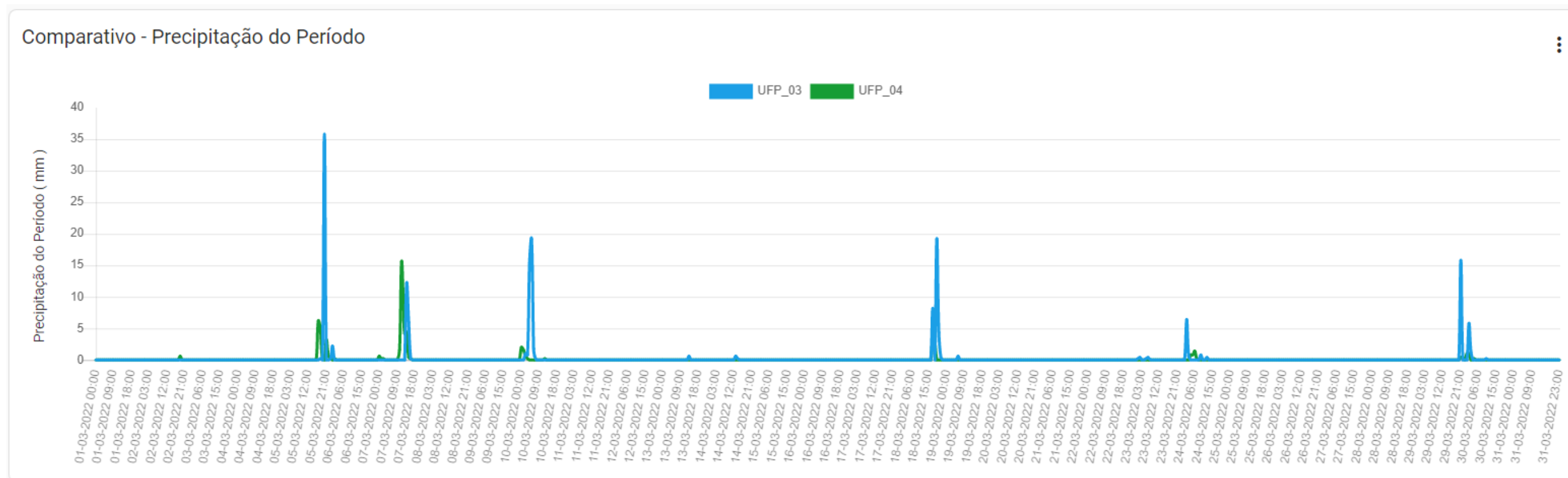
Figura 11 – Precipitação (mm) comparativo nas Estações supracitadas: Estação Barragem-Eclusa (montante) (UFP_03 -Azul) Estação Jaguarão (UFP_04 - Verde)
