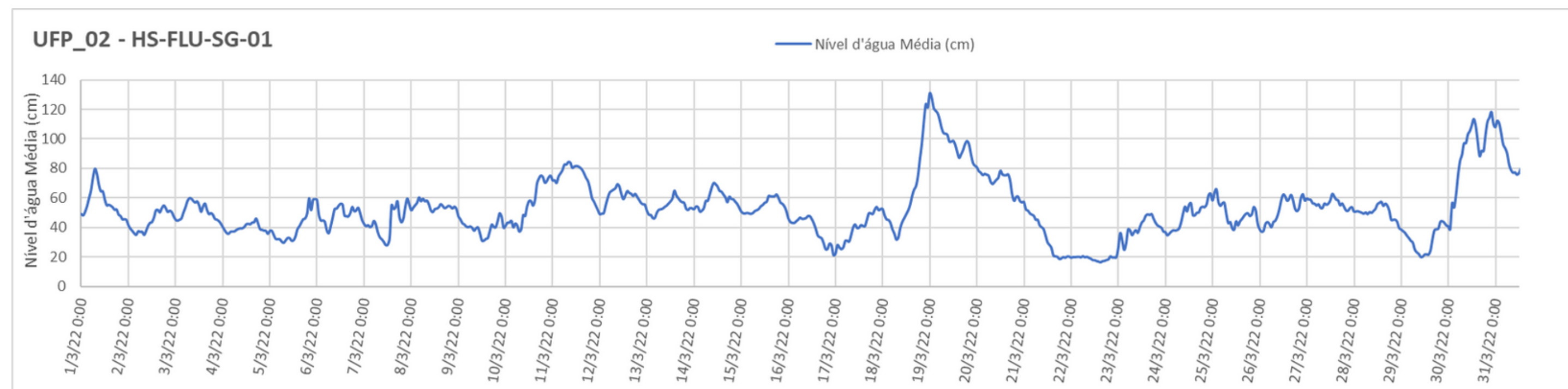
Figura 2 - Nível d'água médio (cm) na Estação Santa Isabel do Sul.
